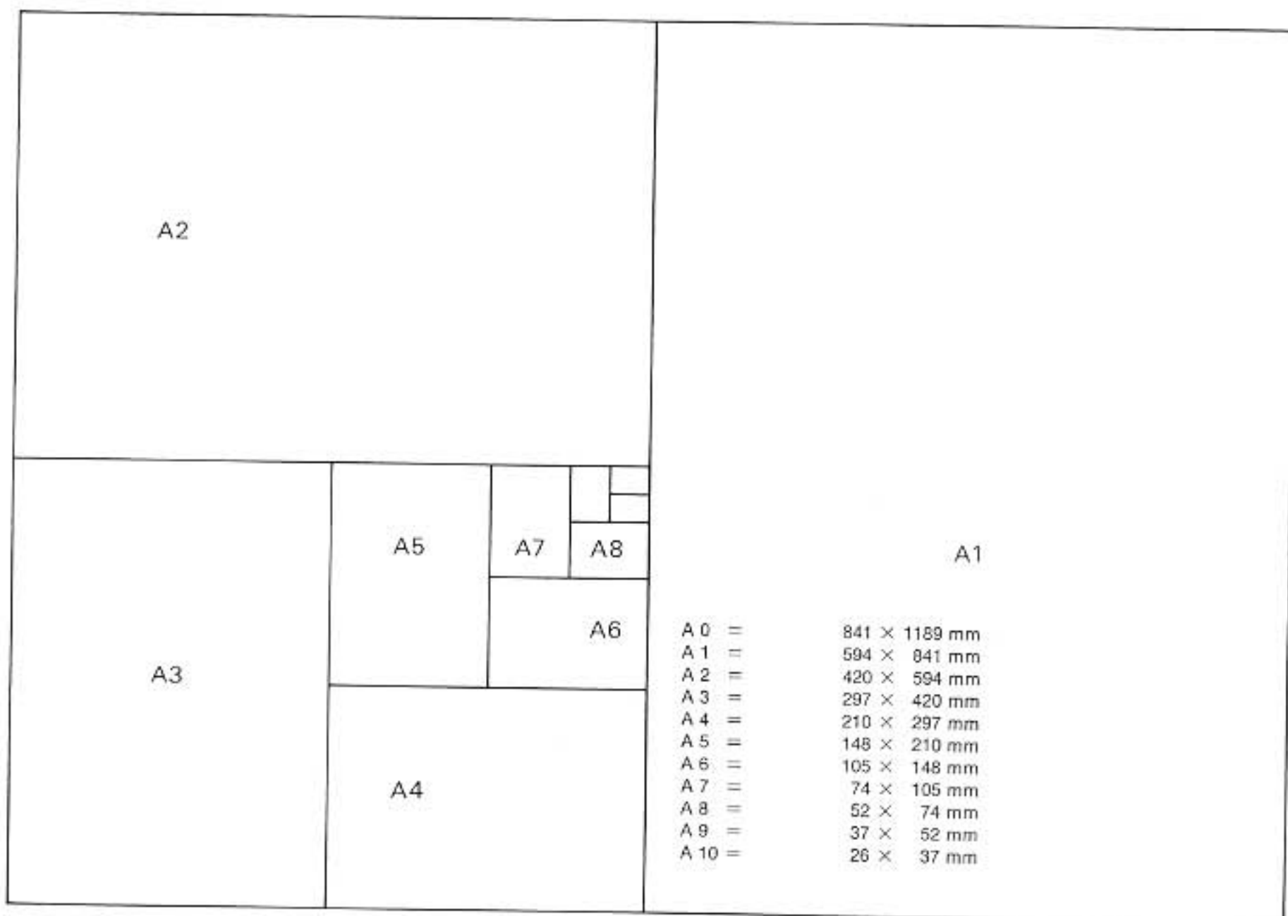
DIN-Formate A 0 bis A 10
