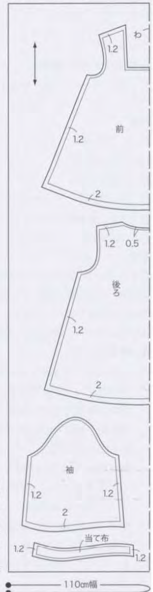
裁合せ図(表布)
