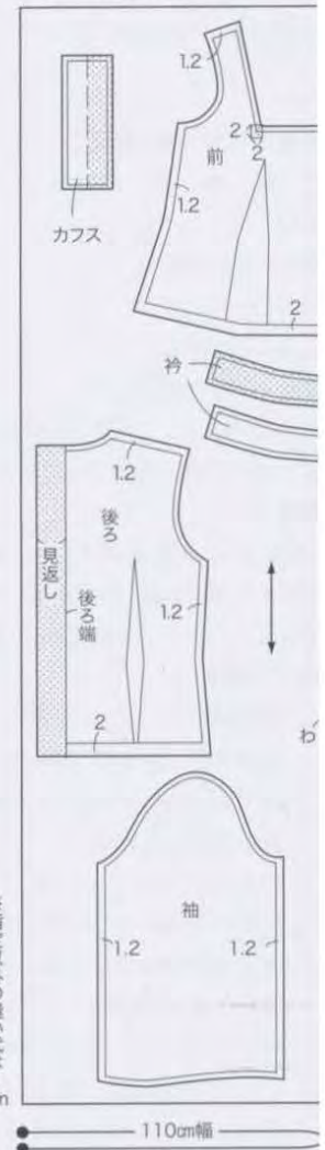
裁合せ図(表布)
